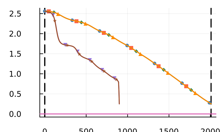
scaled_v
