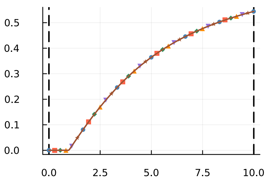
x_3
