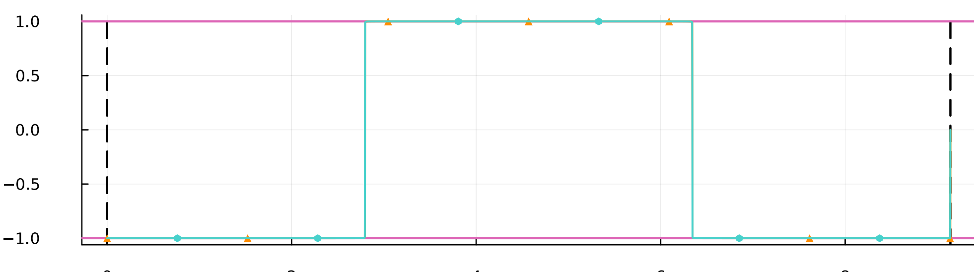
u\phi
